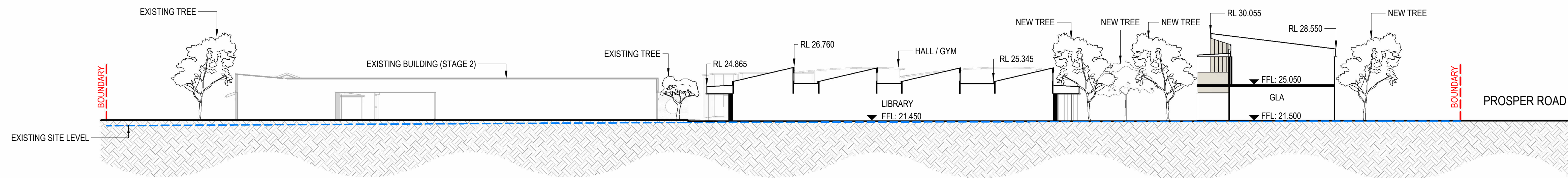
1 SITE SECTION 1 : 250
