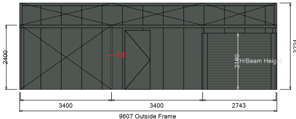
Right Elevation
