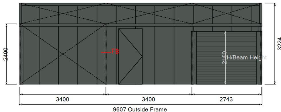
Right Elevation
