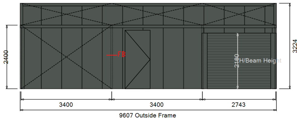
Right Elevation
